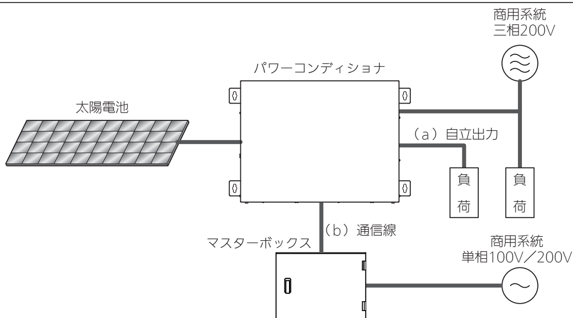
パワーコンディショナ構成図
