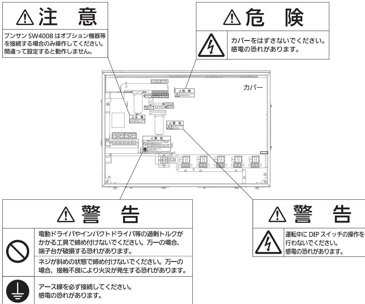
パワーコンディショナ内部配置図
